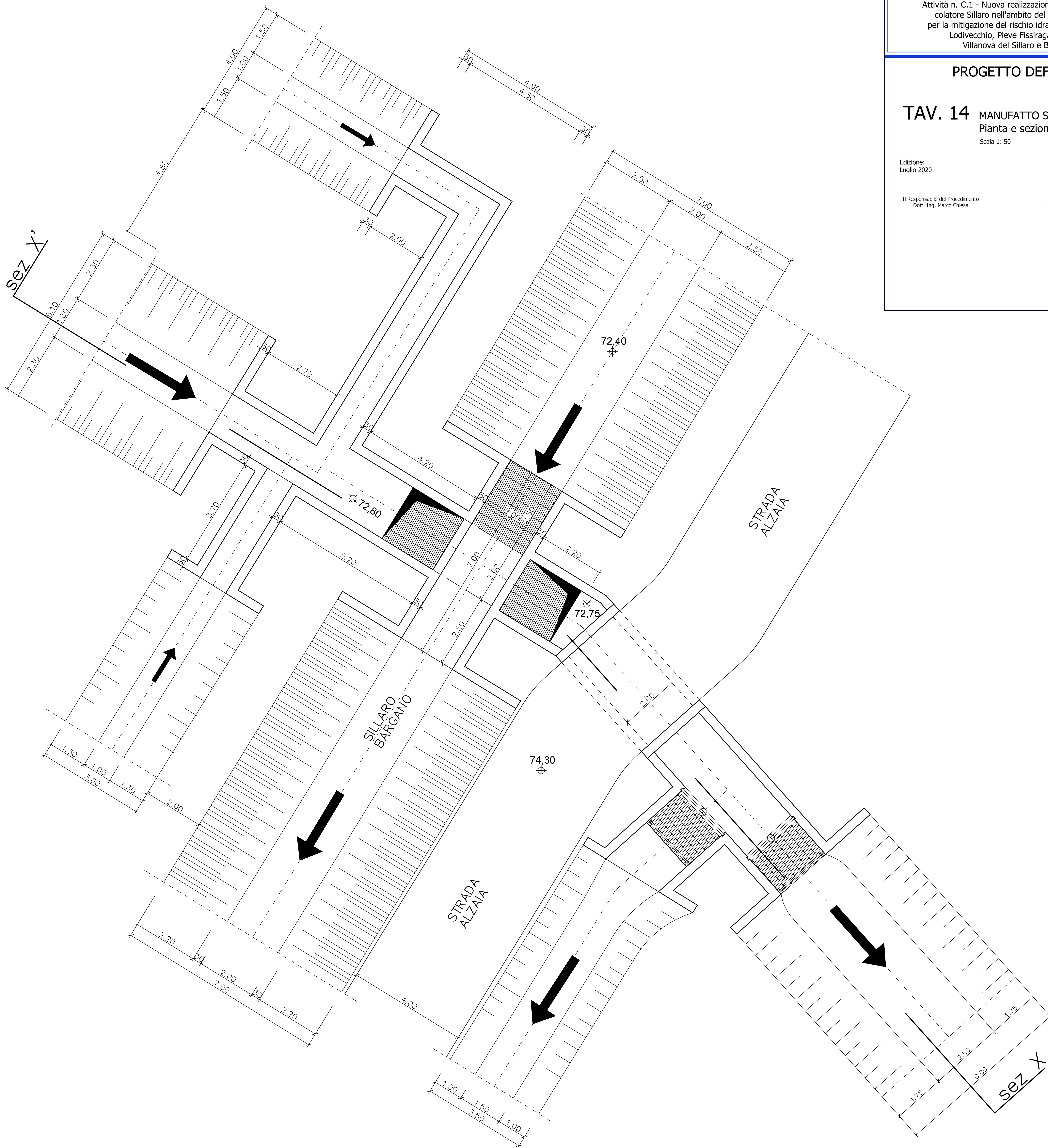
PIANTA MANUFATTO D SIFONE
